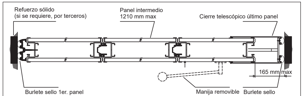
Corte horizontal
